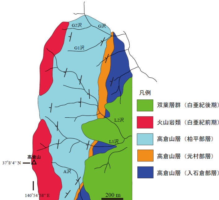
図 1. 八茎地域地質図(Ehiro, 2008 を基に作成).
