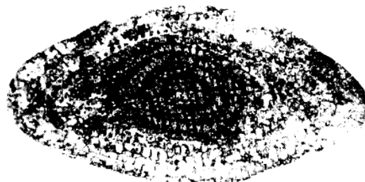
図 10. Colania sp. (Ueno, 1992 より引用)
