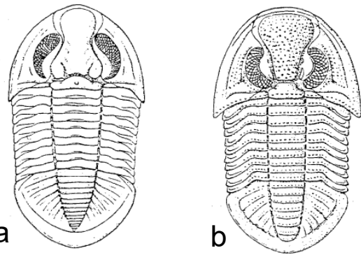
図 6. 高倉山層産三葉虫. (a) Nipponaspis takaizumii , (b) Endops yanagisawai (小林, 1989 より引用).
