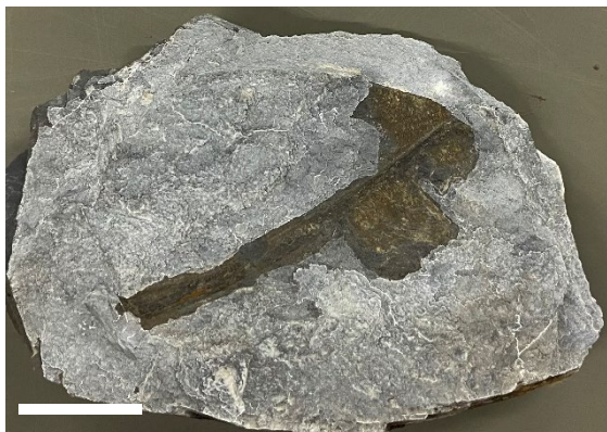
図 9. 柏平部層から産出した植物化石. Taeniopteris sp. (スケールは 5 cm)
