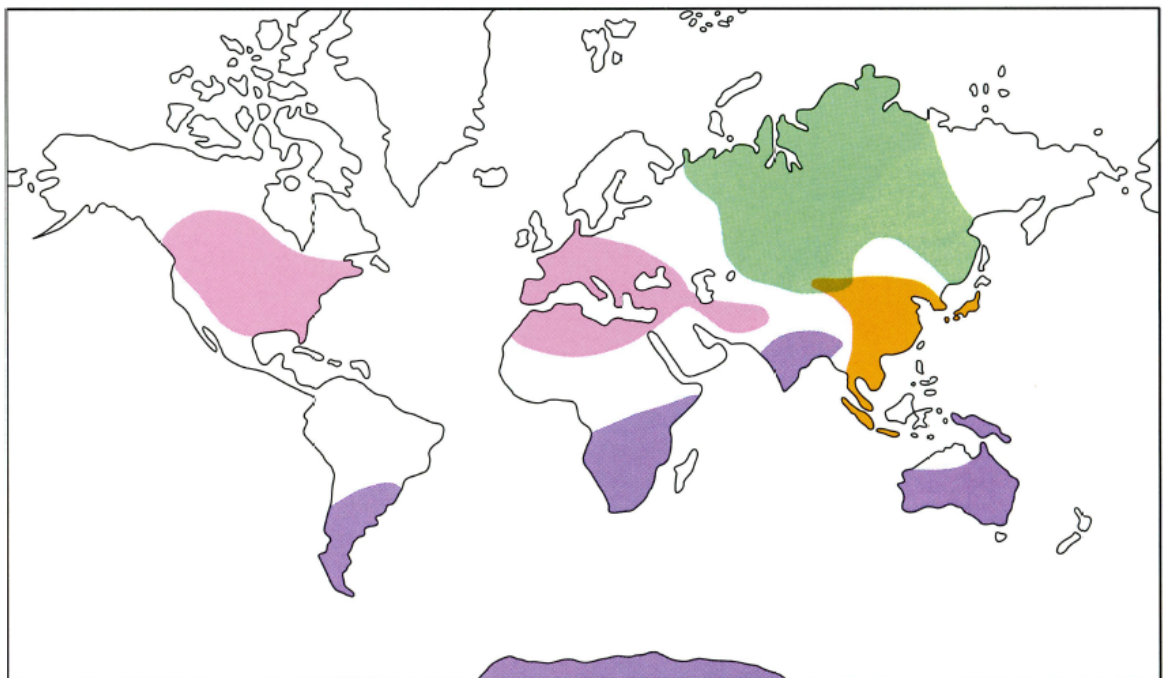
図8. ペルム紀の古植物地理区.
