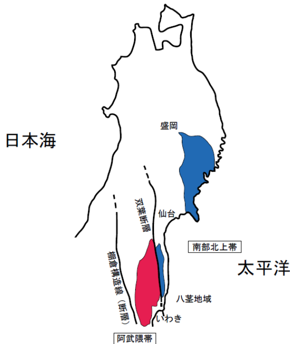
図 3. 南部北上帯及び相当層分布域 (Ehiro, 2008 を基に作成).
