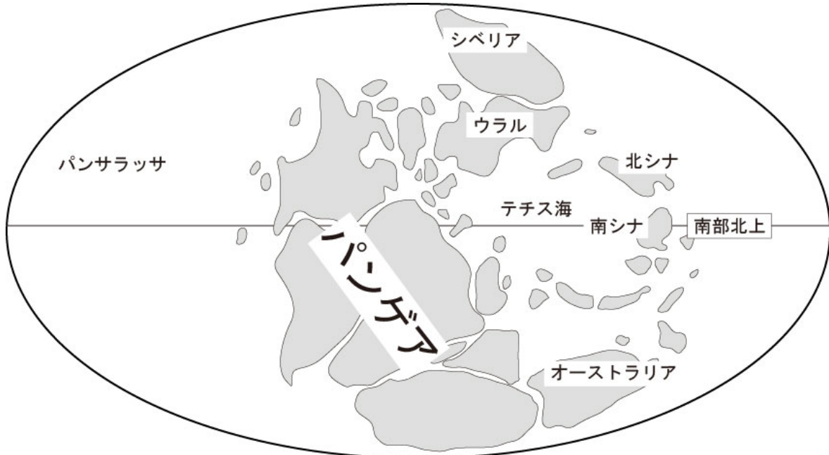
図 11. ペルム紀の古地理図 (永広, 2017a を基に作成).
