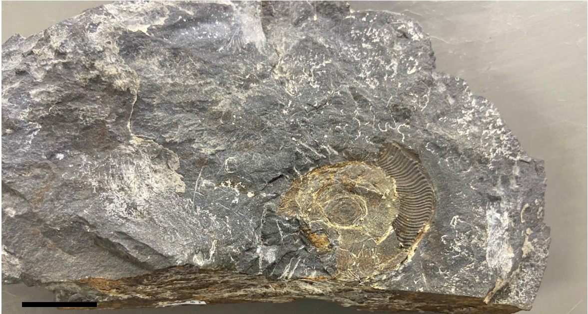
図 4. 柏平部層から産出したアンモナイト化石. Paraceltites sp. (左下のスケールは 2 cm).
